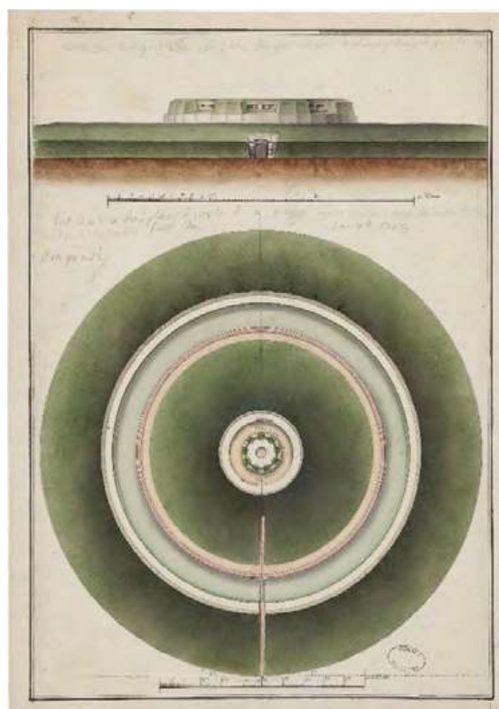
Fonds Montalembert (CP/826AP/15) : plans de forts ronds (fin XVIII e siècle). © Archives nationales de France
