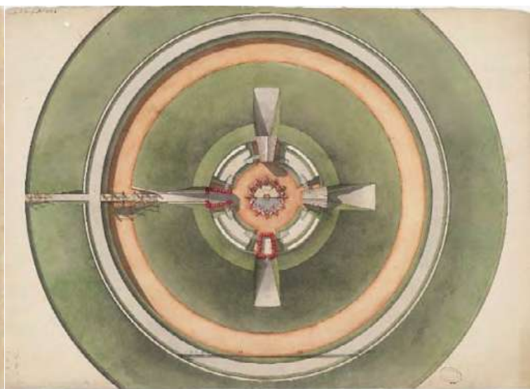
Fonds Montalembert (CP/826AP/15) : plans de forts ronds (fin XVIII e siècle). © Archives nationales de France
