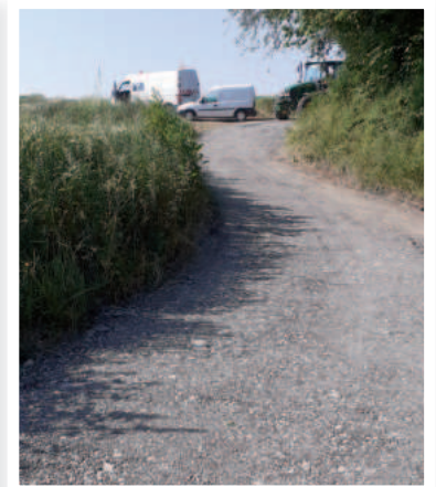
Traitement de chemins ruraux avec matériel de récupération : CAPSO - Coût Commune : 896€
